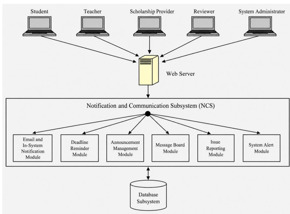
圖十四 NCS 子系統架構圖
